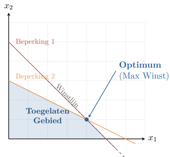
Figuur 6: Grafische oplossing van een LP-probleem
